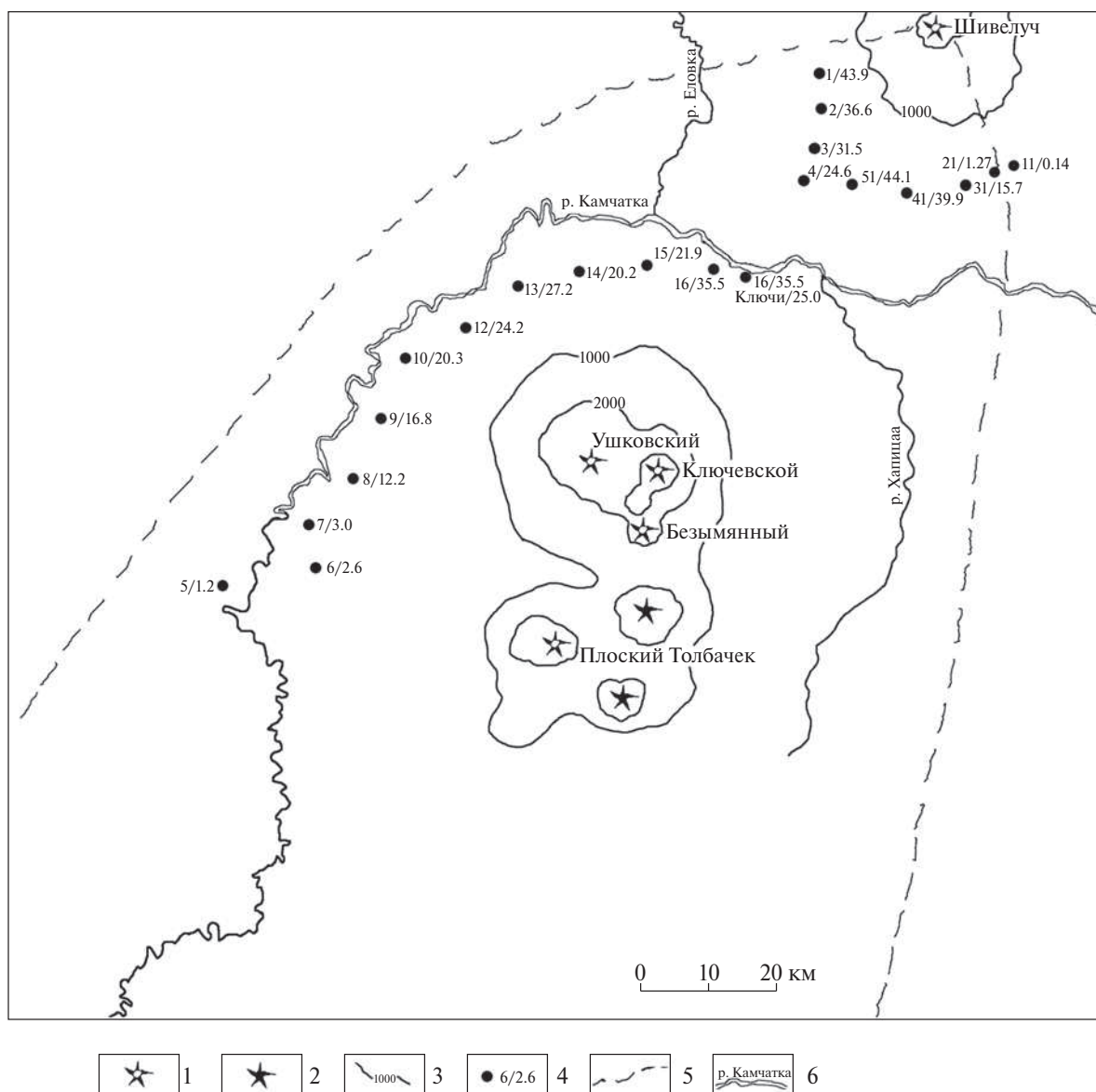
Рис. 7. Схема распространения пепловых отложений и мест отбора проб пепла извержения вулкана Шивелуч 11.04.2023 г.
