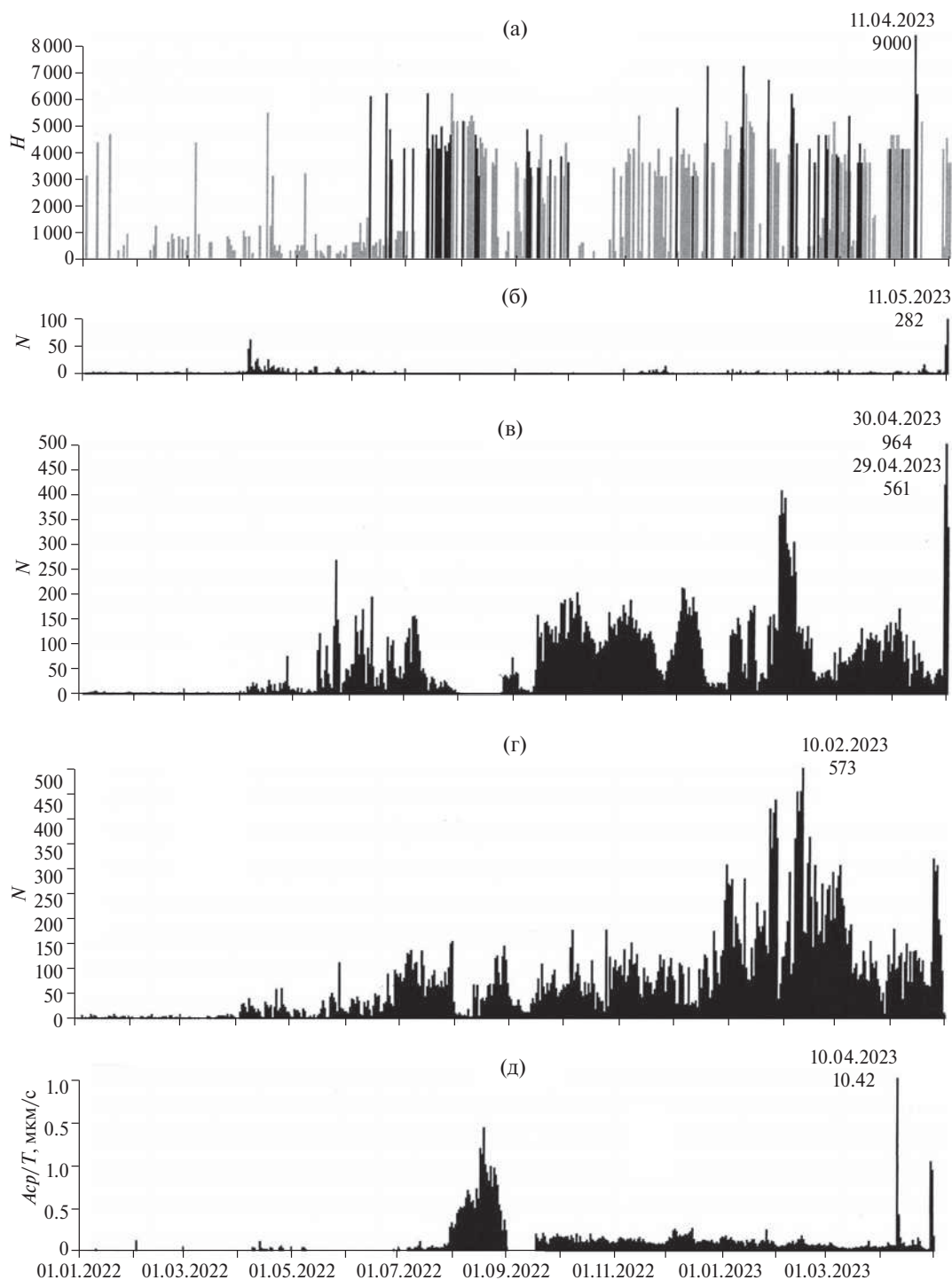
Рис. 2. Суточные характеристики сейсмической и вулканической активности в 2021–2023 гг.
