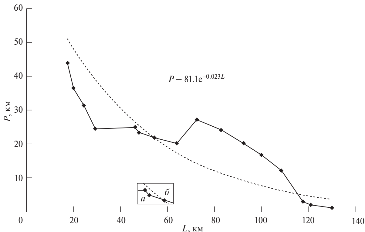
Рис. 6. График убывания пепловых отложений во время катастрофического извержения вулкана Шивелуч 11.04.2023 г.
