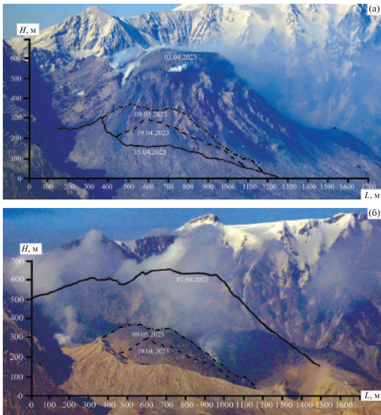
Рис. 3. Профили лавового купола до извержения (а) и после извержения (б) вулкана Шивелуч 11 апреля 2023 г.
