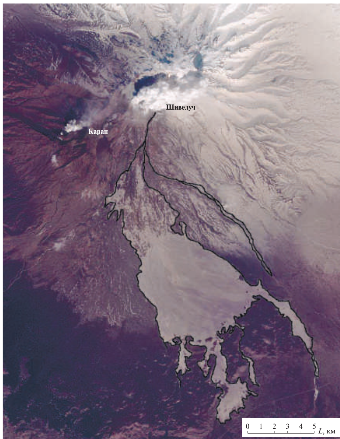
Рис. 5. Схема отложений продуктов направленного взрыва во время катастрофического извержения вулкана Шивелуч 11 апреля 2023 г.
